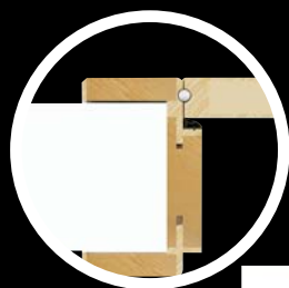
B) DVERE A ZÁRUBŇA BEZFALCOVÁ
