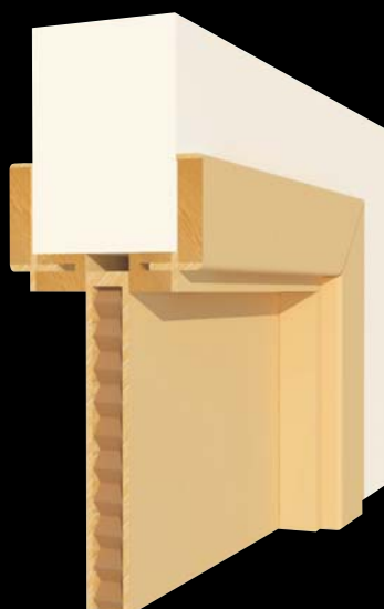
B) REZ OBLOŽKOU PRE STAVEBNÉ PÚZDRA A DVEREMI (VOŠTINA)
